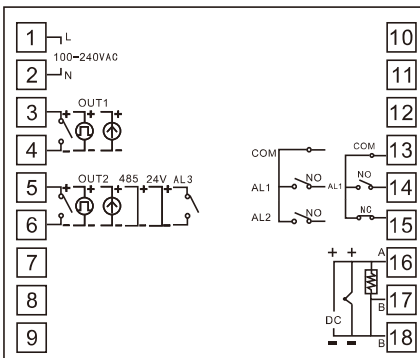
3.1、MG904接线图(标准)
