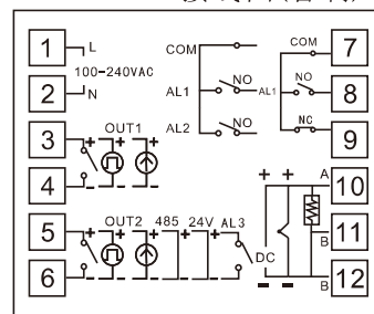
3.2、MG904接线图(客制)
