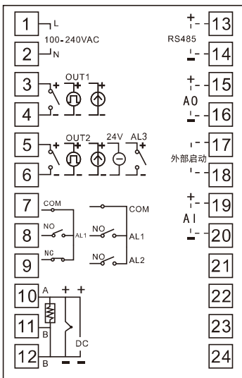
1、MG909与MG908接线图
