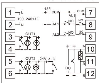
3.1、MG904接线图(标准)
