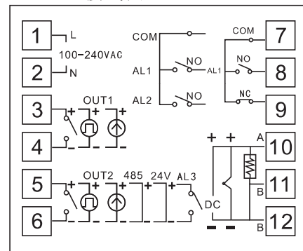
3、MG904接线图
