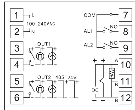
3、MG904接线图
